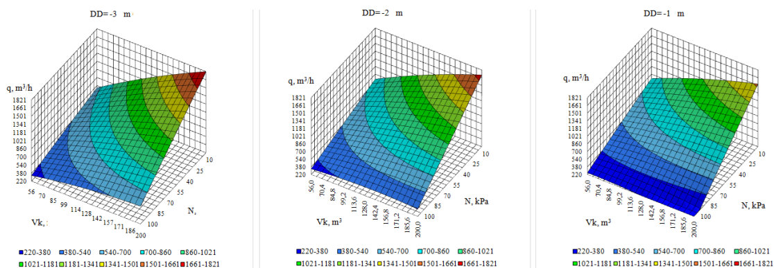
Фигура 1. Изолинии за максимална почасова производителност в околността на оптимума при всички комбинации на факторите, за плавателния съд Hopper Dredger "GLANFORD".
